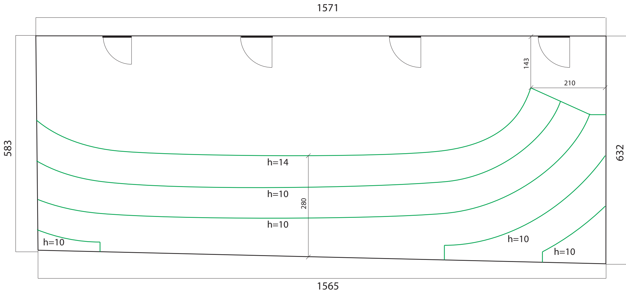
SCHODY DO ROZBIÓRKI - SCHEMAT
